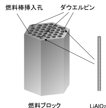
図 2 \text{LiAlO}_2 の装荷
