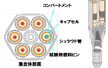
照射燃料集合体 (B型)
