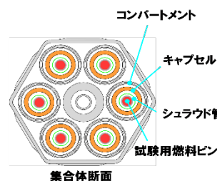
照射燃料集合体 (B型)
