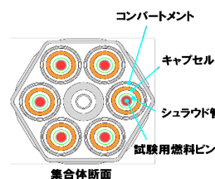
照射燃料集合体 (B型)
