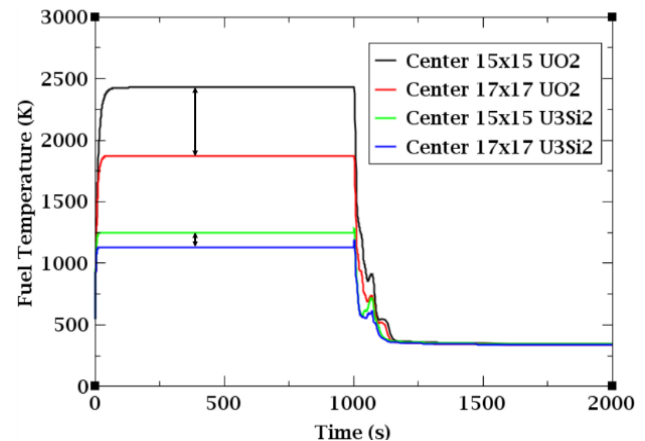
図 1 LOCA 時の燃料棒最高温度
