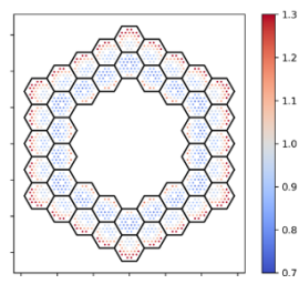
図4 径方向出力分布 (サイクル末期)
