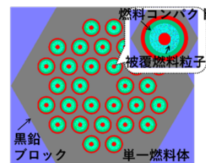
図1 高温ガス炉燃料体
