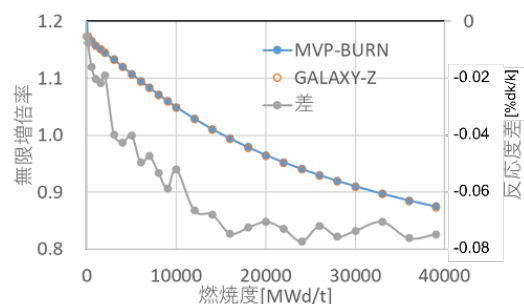
図2 MVP-BURN との比較
