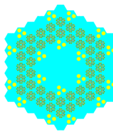
図3 高温ガス炉 環状炉心
