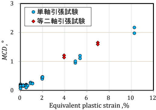
図 2 相当塑性ひずみと方位差の関係
