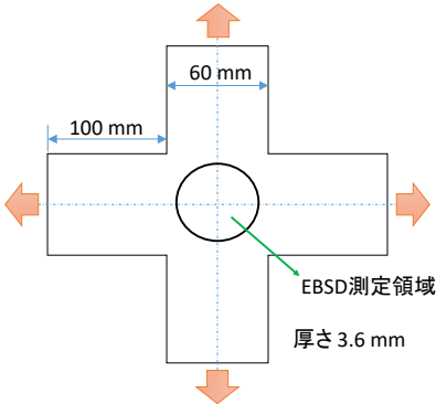
図 1 十字試験片を用いた等二軸引張試験
