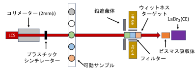
図 1 UVSOR での 1 次元イメージング実験の配置図
