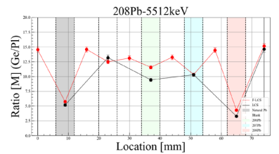
図 2 208 Pb の NRF レベル (5512 keV) を用いた 1 次元イメージ (赤線 : F-LCS ガンマ線、黒線 : LCS ガンマ線)
