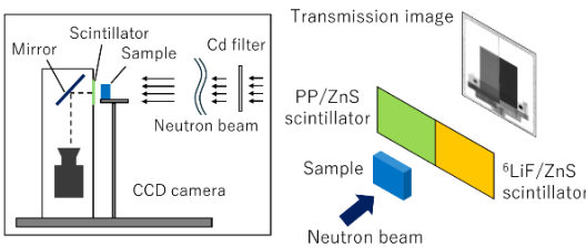
図 1 撮影体系の概略図
