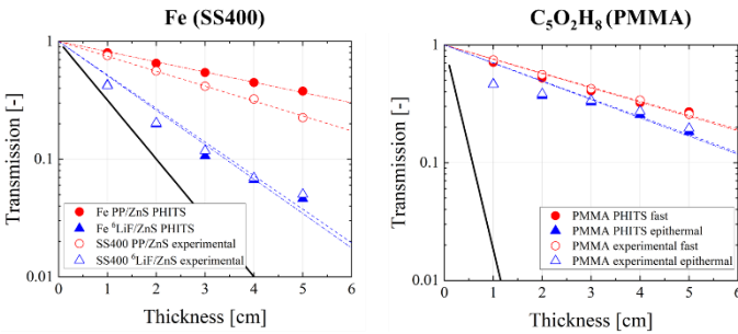
図 2 6 LiF/ZnS、PP/ZnS シンチレータによる透過像における水平方向の透過率の比較
