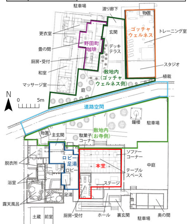
図-1 西圓寺の施設配置図
