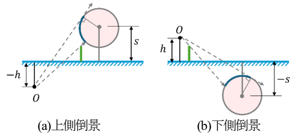
図-13 倒景の計算方法
