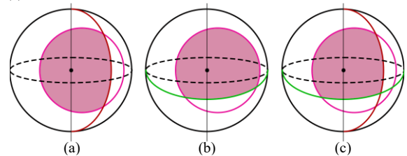
図-17 球帽を切り取る隣接平面と草木平面
