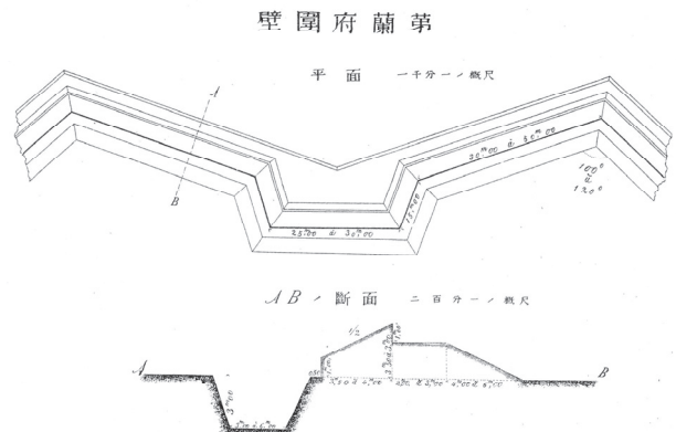
図 6: 古川による稜堡式城壁実測調査図(出典:文献 25)
