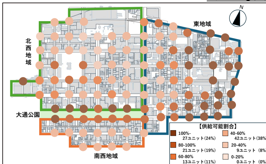
図3-4. 各ユニットにみる再エネの供給可能割合
