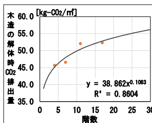
図 3-8. 木造の解体時 CO 2 排出量
