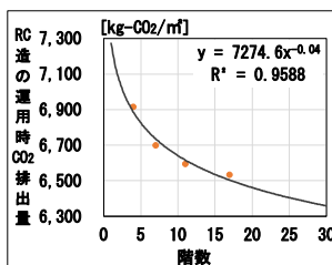
図 3-6. RC 造の運用時 CO 2 排出量
