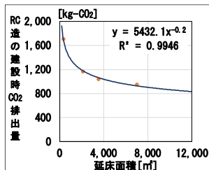
図 3-4. RC 造の建設時 CO 2 排出量
