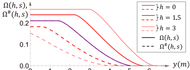
図-15 視点高の感度分析
