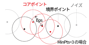
図 5. DBSCAN の仕組み
