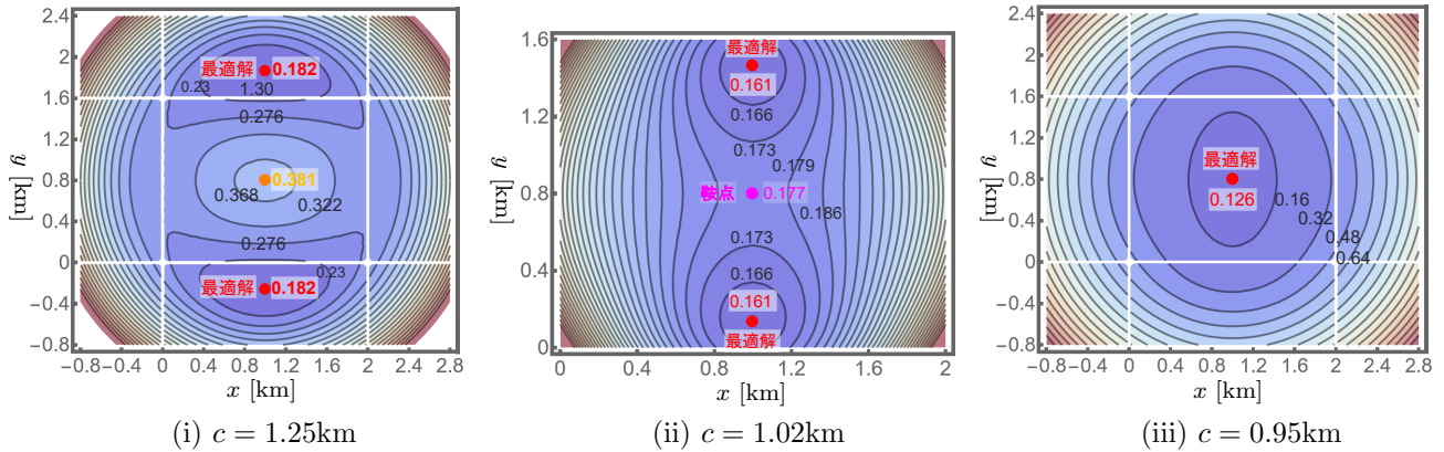
図3 (L, M) = (2\text{km}, 1.6\text{km}) の矩形領域における一様な人口分布の下での理想徒歩距離からの乖離の2乗の平均値 f(x, y) の等値線 ( k = 0.5 の場合)。
