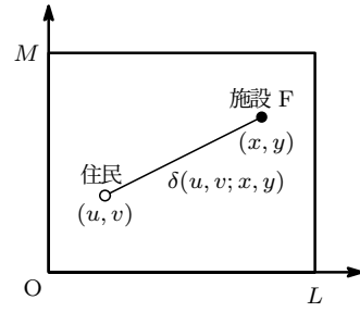
図 1 L \times M の矩形都市領域内の単一施設と住民。
