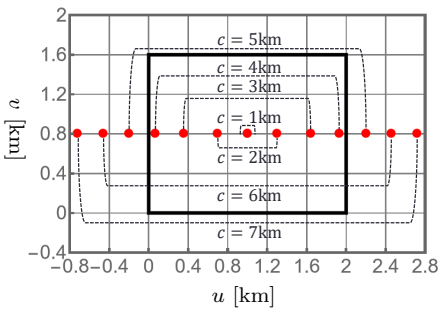
図9 施設数 \nu = 2 での h の最小解 ( k = 1 , c = 1\text{km} \sim 7\text{km} )
