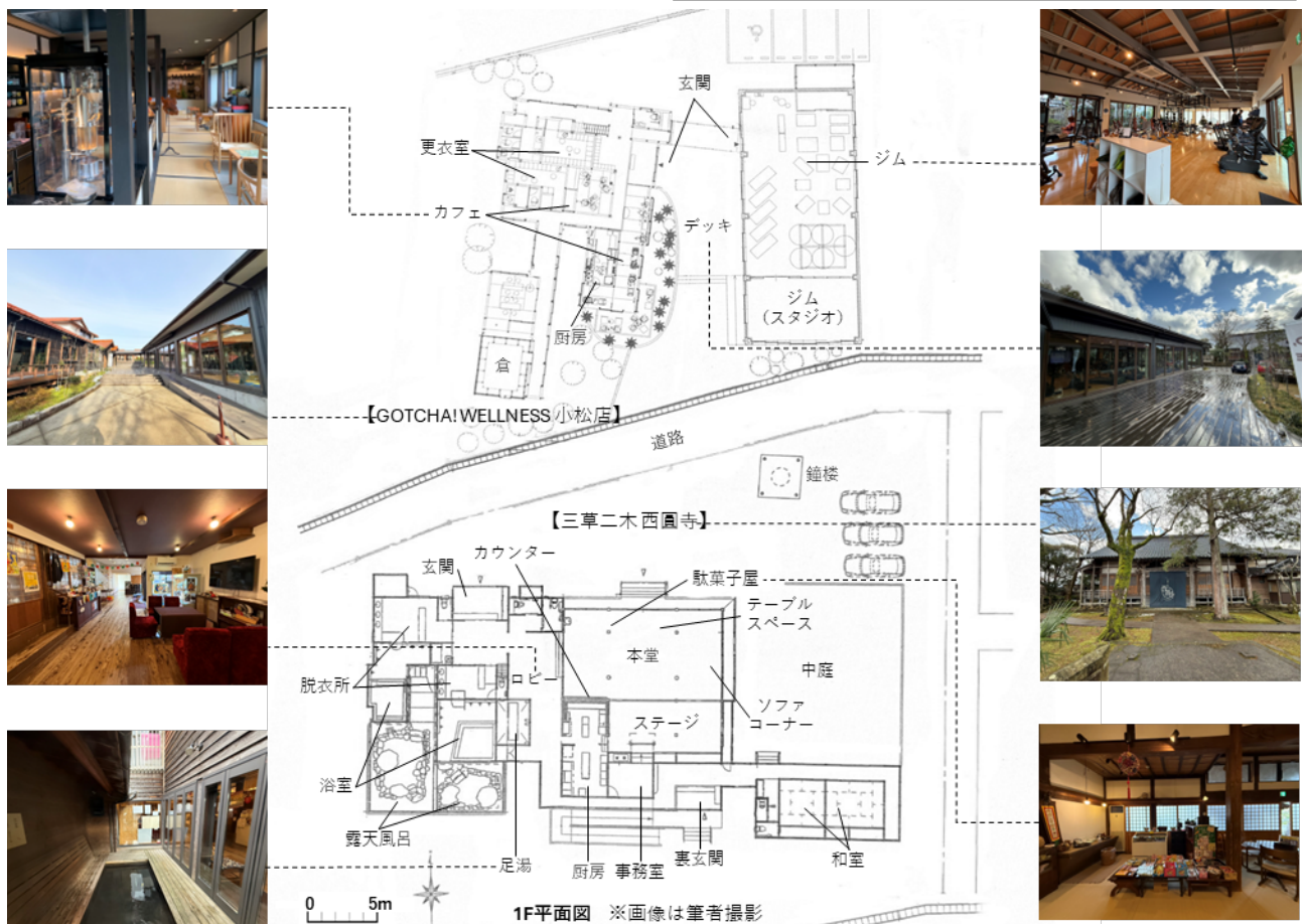
図-1 西圓寺 1 階平面図
