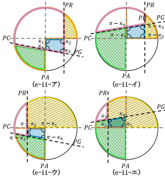
図-19 4平面で定まるV字切断面
