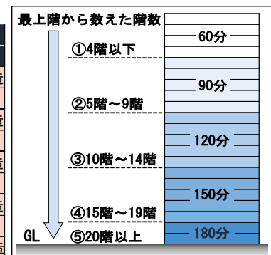
図 3-1. 階層別耐火時間
