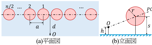
図-4 配置図
