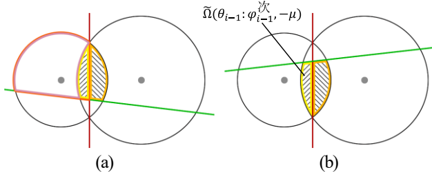
図-20 隣接平面と草木平面との交わりでの立体角
