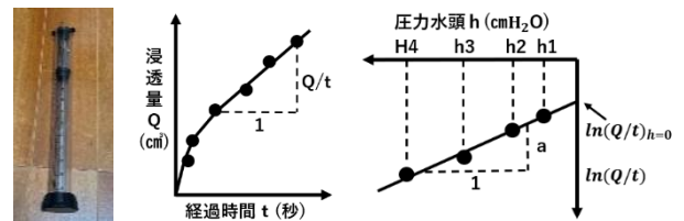
図7. インフィルトロメータ(左図) 18)
