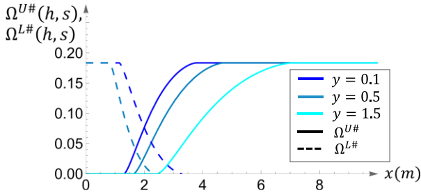
図-14 草木繁茂と上側・下側倒景立体角
