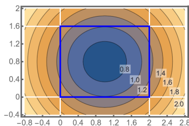
図 A3 (L, M) = (2, 1.6) の一様な矩形盤から施設点への平均距離の等値線 (矩形盤の境界を図中の青い線で表している)。
