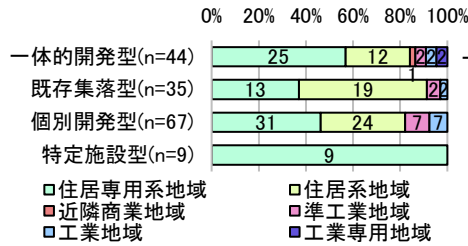
図-6 最も広く隣接する用途地域との関係
