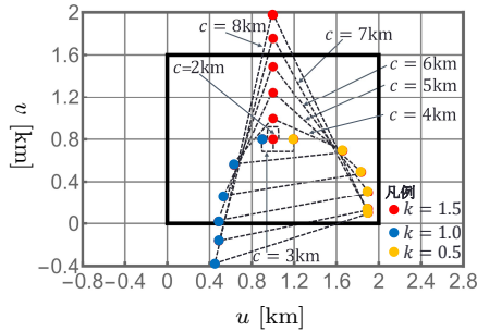
図8 施設数 \nu = 3 のでの g の最小解 ( \{k_1, k_2, k_3\} = \{1.5, 1.0, 0.5\} , c = 2\text{km} \sim 8\text{km} ).
