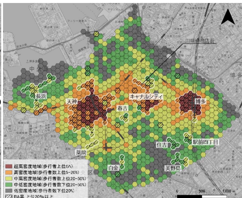
図-5 歩行者数による地域区分と高 RA 率地区
