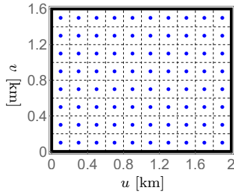
図4 矩形領域内で居住者の点を格子状に与える様子。 (( L, M ) = (2km, 1.6km) で、格子点間隔は 0.2km)
