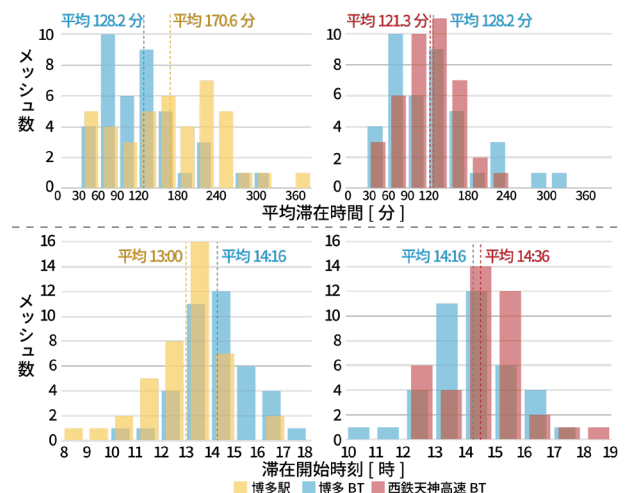
図 7. 滞在ポイントの数が上位 40 位のメッシュにおける平均滞在時間・滞在開始時刻の分布
