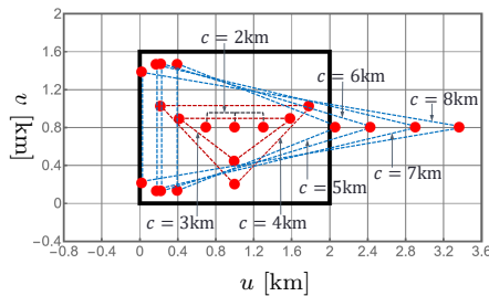
図10 施設数 \nu = 3 での h の最小解 ( k = 1 , c = 1\text{km} \sim 8\text{km} )
