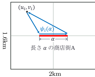
図12 点 (u_i, v_i) を出発し 2\text{km} \times 1.6\text{km} の地域中央の長さ \alpha の商店街を訪れて帰宅する巡回距離 \psi_i(\alpha) .
