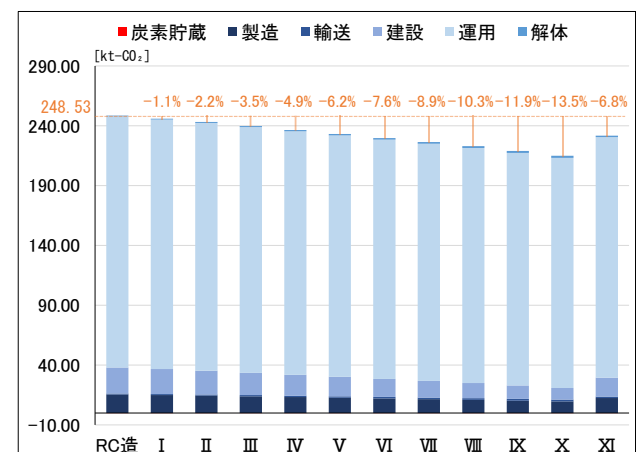
図 3-9. RC 造と木造の LCCO 2 と削減率
