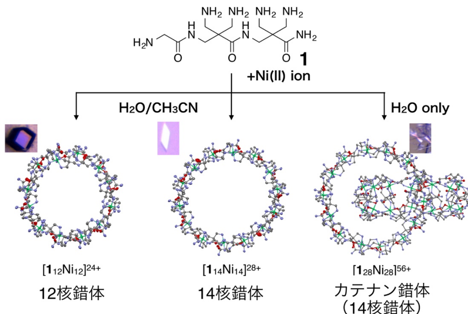
図 1. トリペプチド 1 から形成する 3 種類の巨大環状錯体の構造とその形成条件
