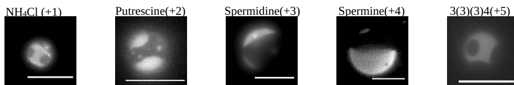
Fig1. DOPS/DPPC/Chol からなるリポソームに塩添加での相分離画像(Scale bar :10 μm)
