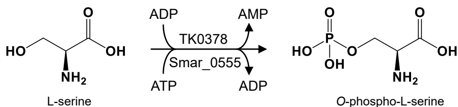
図 1. Serine kinase が触媒する反応
