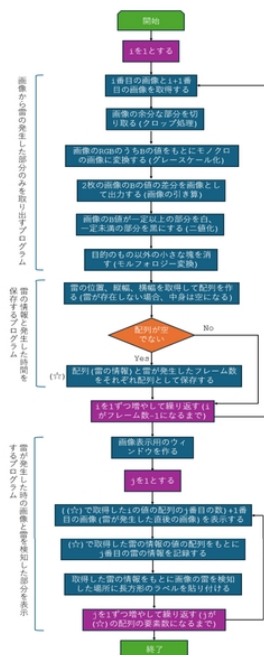
Fig4. 動画解析プログラムのフローチャート
