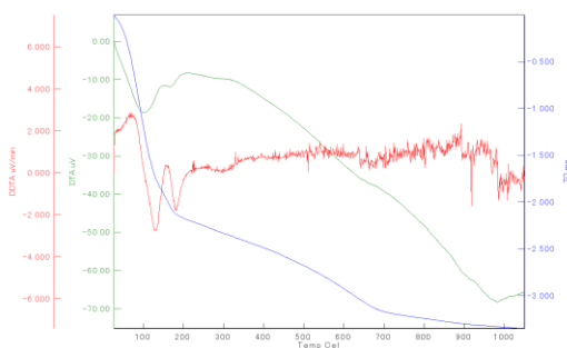
Fig 1. 軽石質火山礫凝灰岩を水鋏処理した試料の示差熱分析結果。DTA 曲線(緑)は 100-200・600・900-1000°C付近に吸熱反応を示すピークが認められバーミキュライトと類似する。
