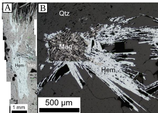
Fig. 1: 鉄鉱石の反射顕微鏡写真 (A) 一部磁鉄鉱化した針状赤鉄鉱。花崗岩の distal skarn 中の鉱体（帯磁率： 520 \times 10^{-3} SI）でみられる。 (B) 赤鉄鉱がオーバーグロースした磁鉄鉱。ドレライトの proximal skarn 中の鉱体（帯磁率： 200 \times 10^{-3} SI）でみられる。〈Hem: 赤鉄鉱, Mag: 磁鉄鉱, Qtz: 石英〉
