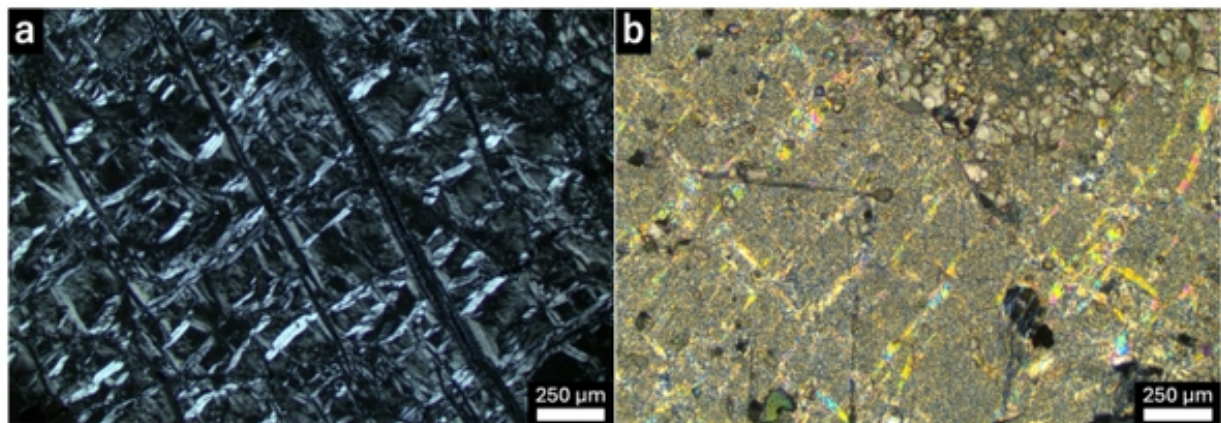
Fig. ブロック部の蛇紋岩(a)と滑石-炭酸塩岩(b)のメッシュ組織の偏光顕微鏡写真(クロスニコル)
