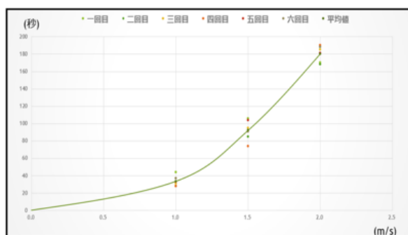
図 ループリング型を用いた実験結果
