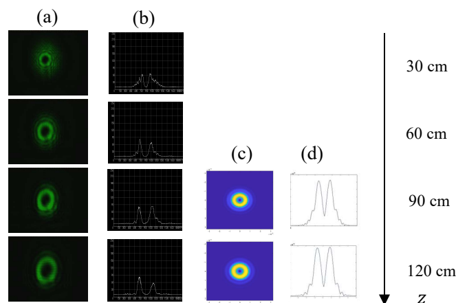
Fig. 2: SLM で生成した高次光子 (a) 空間強度分布 (実験) (b) 断面強度分布 (実験) (c) 空間強度分布 (シミュレーション) (d) 断面強度分布 (シミュレーション)
