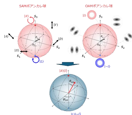
図 1 : 高次ポアンカレ球
