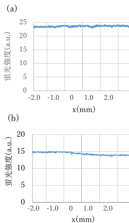
図 1. キャピラリー軸方向の量子ドット密度分布, x = 0 が電場極大位置. (a)測定開始時, (b)測定開始から 4 時間後
