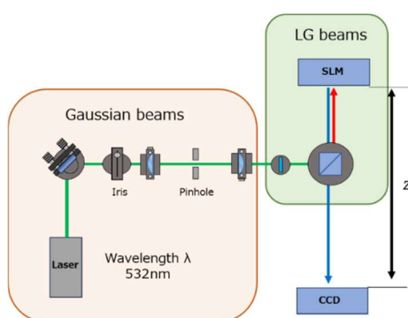
Fig. 1: SLM を用いた高次光子生成のための光学系。
