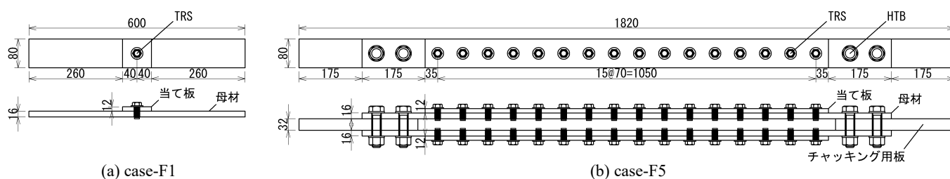
図-1 疲労試験体
