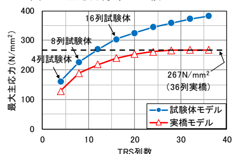
図-5 TRS 列数と最大主応力との関係
