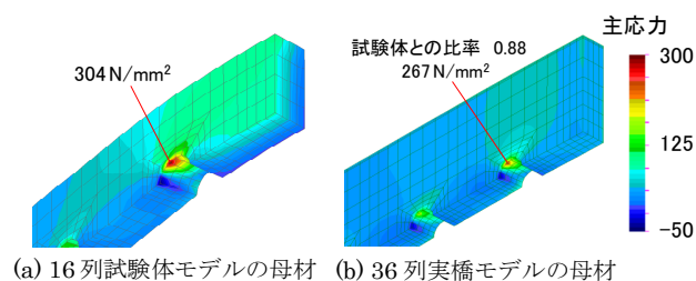
図-4 主応力分布の比較
