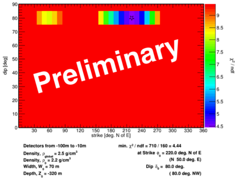
図 2:断層を 1 枚板であると仮定した場合に最も観測データと一致した断層のパラメータと、走行-傾斜平面における \chi^2 乗/自由度の様子
