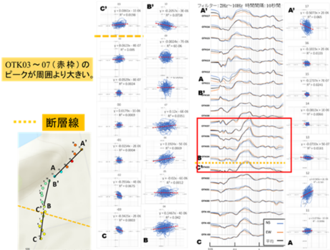
大塚地区の断層近傍のH/Vと粒子軌跡
