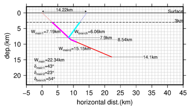
図2 統計的グリーン関数法による地震動評価に用いた 断層モデル断面図 赤線は主断層、ピンク色は主断層のアスベリティ、 青線は分岐断層を、水色は分岐断層のアスベリティ
