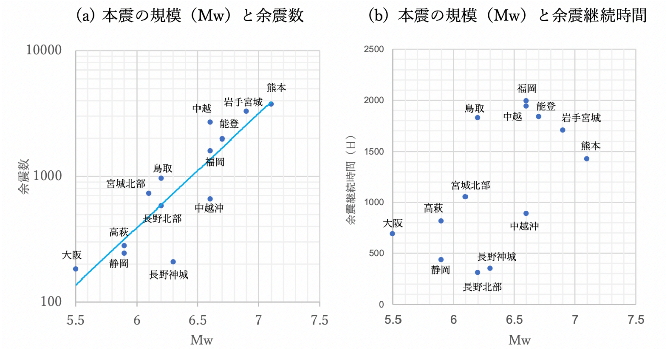
図 1 . (a)余震数および(b)余震継続時間と本震の規模の関係。(a)内の水色直線は、余震数が地震の規模の 1 次関数として表されると仮定した際に、最小二乗法により求められた回帰直線を示す。
