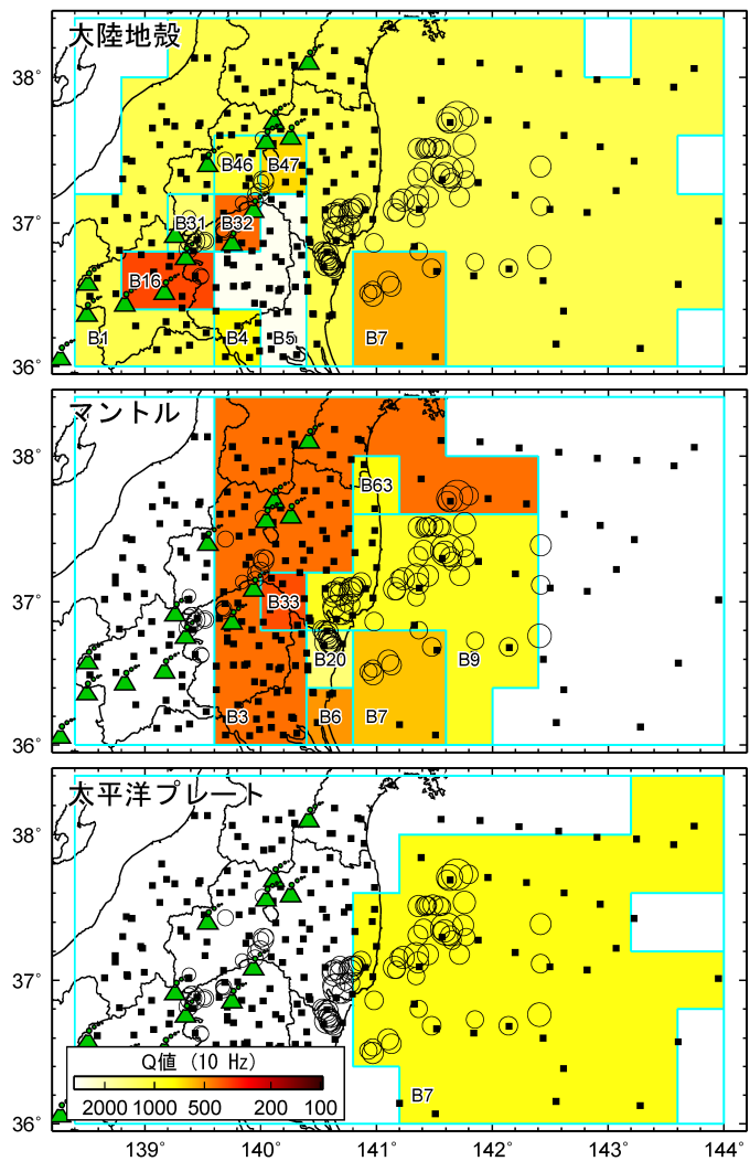
図 3 推定した不均質減衰構造 (カラーは 10 Hz の Q 値)
