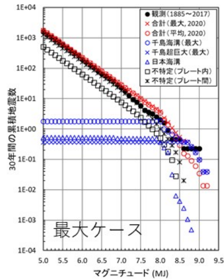
太平洋プレート地震
