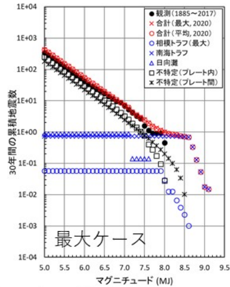
フィリピン海プレート地震
