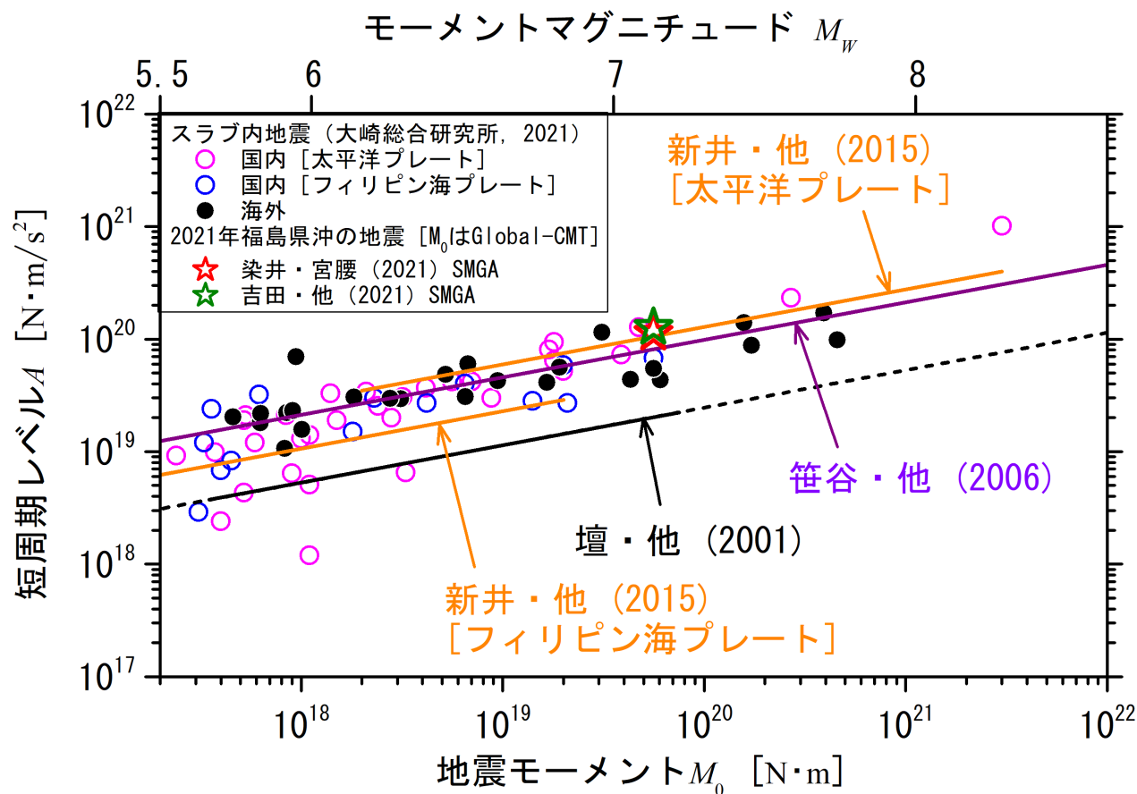
図1 スラブ内地震の地震モーメントと短周期レベルの関係 (暫定結果)
