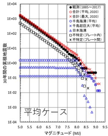
太平洋プレート地震
