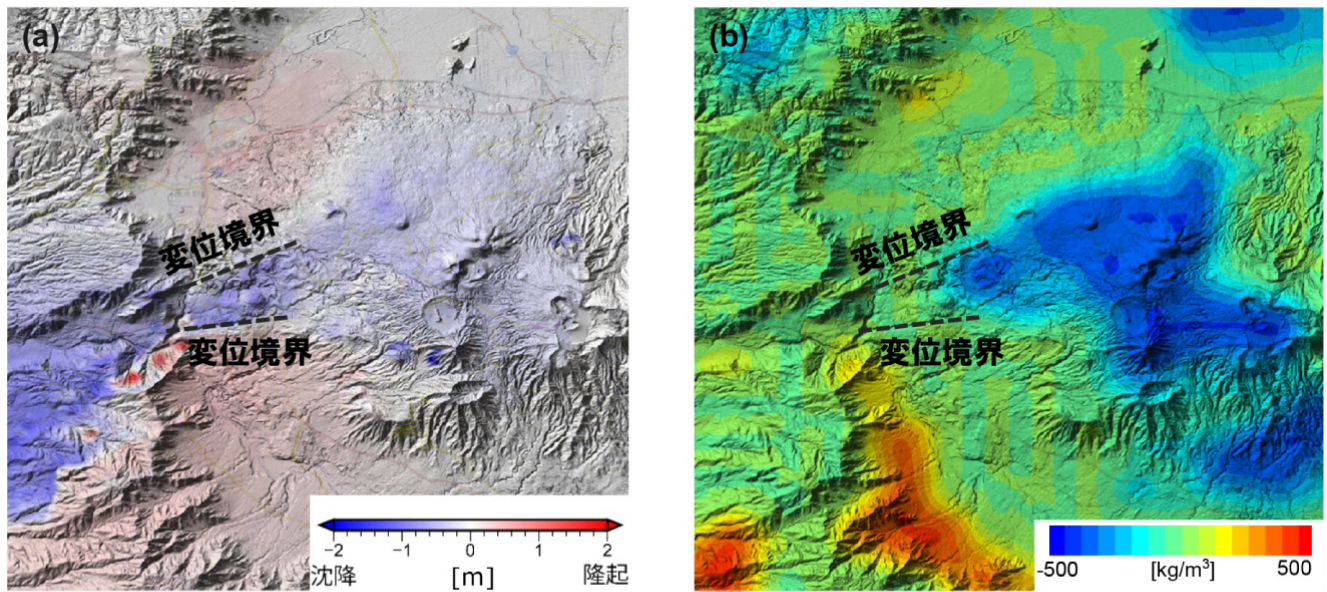
図1 (a) 干渉SAR解析から得られた上下変位. (b) 重力インバージョンによって推定された阿蘇カルデラ西縁周辺の地下密度不均質構造(深さ1.5kmの水平断面). 青色(赤色)は周囲よりも密度が低い(高い)領域を表す.
