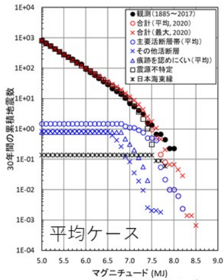
陸側プレートの浅い地震
