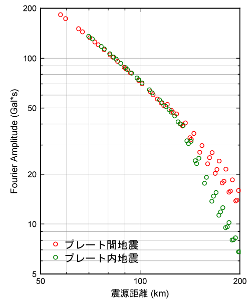
図 5 距離減衰特性の比較 (10 Hz)
