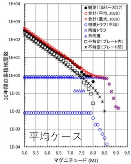
フィリピン海プレート地震
