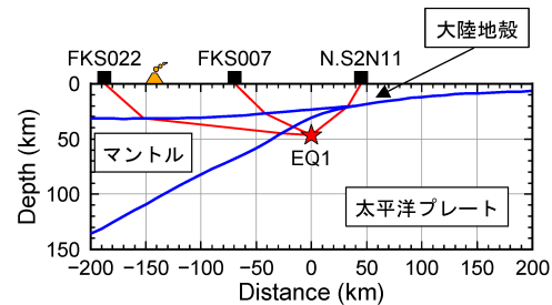
図 2 2次元レイトレースの例
