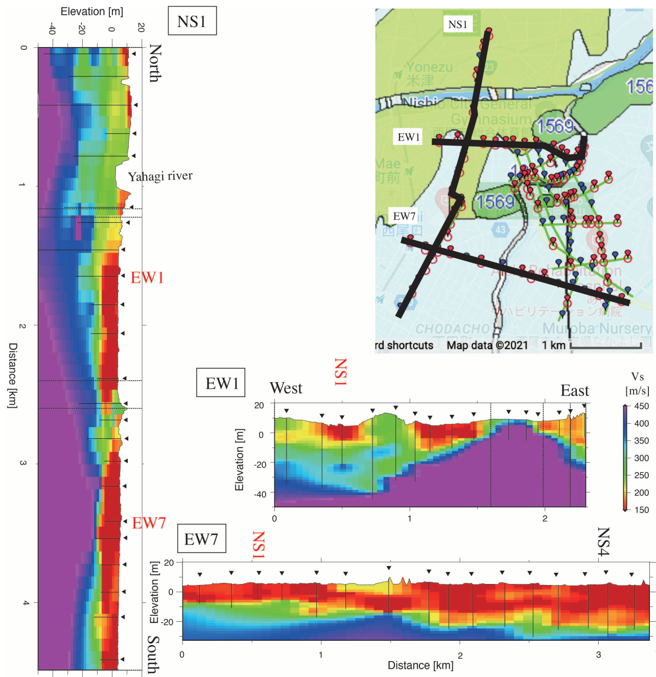
図1 測線沿いのVs構造鉛直断面(測線NS1, EW1, EW7). 右上の地質マップの太線は測線位置を示す. 速度断面の縦点線は測線の折れ曲がる箇所, 三角は観測点位置, 三角直下の縦棒は速度構造モデルの最下層までの深さを示す.
