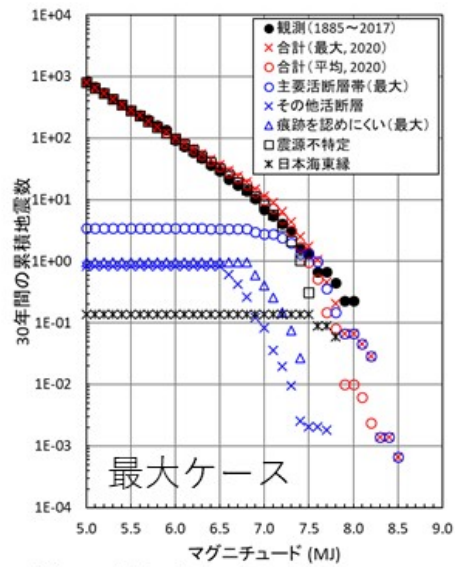
陸側プレートの浅い地震
