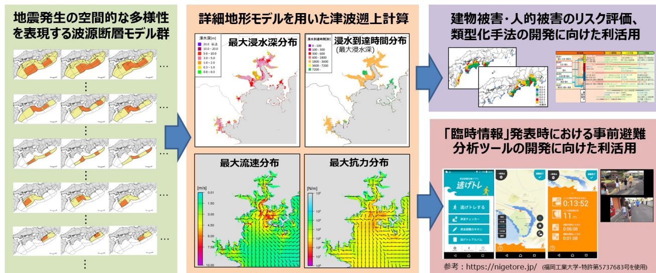
図1 本研究の概要。本研究では、南海トラフ巨大地震に対する空間的な多様性を表現する膨大な数の波源断層モデル群（図左側）を用いた津波遡上計算を実施し、多様な津波ハザード情報を創出する（図中央）。創出する津波ハザード情報について、建物被害・人的被害等のリスク評価、南海トラフ巨大地震の地震像に対する類型化手法の開発、「臨時情報」発表時における事前避難分析ツールの開発に向けた利活用等を想定している（図右側）。
