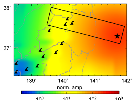
図 4 基盤面上の 10 Hz の距離減衰特性の面的分布 (プレート内地震)
