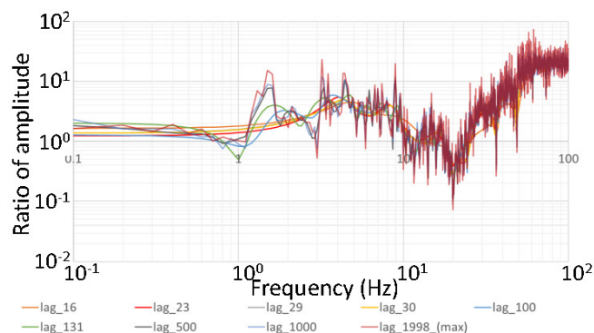
図3. ARモデルのスペクトルで見た地表/地下の振幅比の次数による違い
