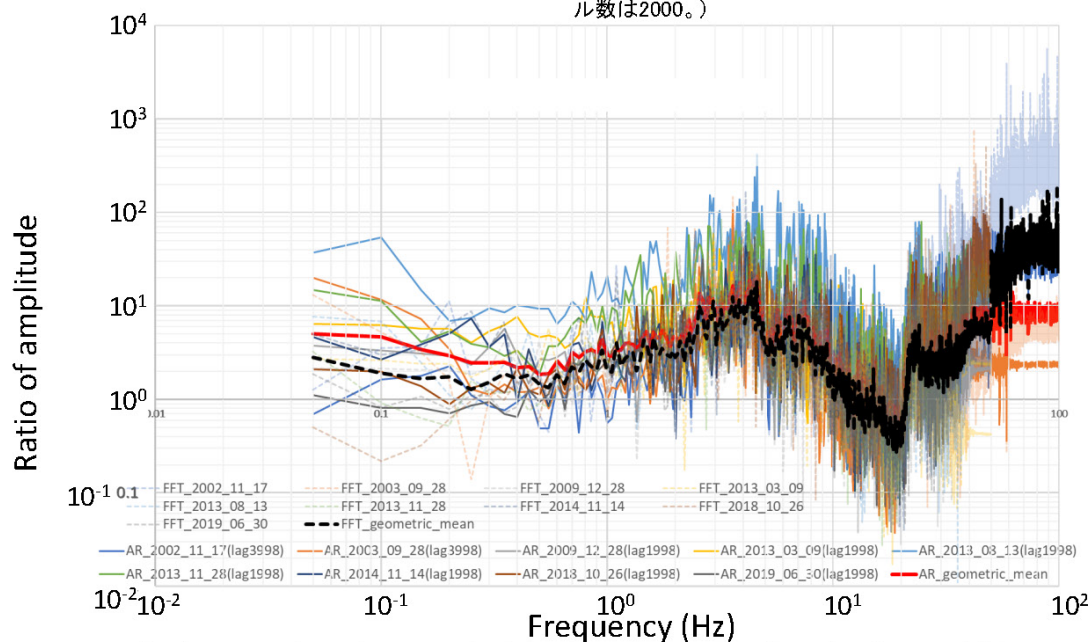
図4. ARモデルとFFTによるスペクトルで見た地表/地下の振幅比の比較(S波20秒間NS成分)
