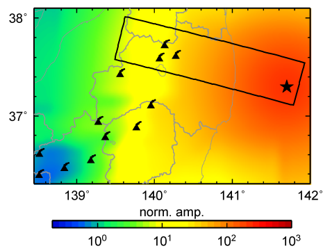
図 4 基盤面上の 10 Hz の距離減衰特性の面的分布 (プレート内地震)
