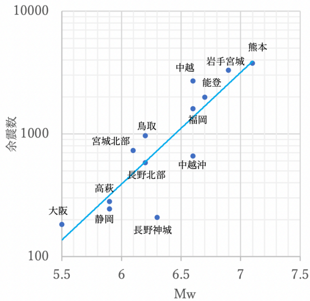
図1. (a)余震数および(b)余震継続時間と本震の規模の関係。(a)内の水色直線は、余震数が地震の規模の1次関数として表されると仮定した際に、最小二乗法により求められた回帰直線を示す。
