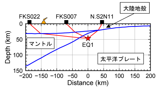
図 2 2次元レイトレースの例
