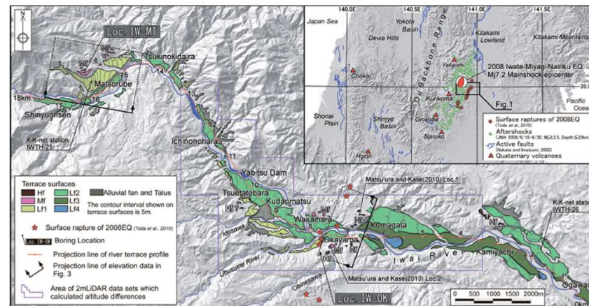
図1 段丘面区分図および調査位置図
