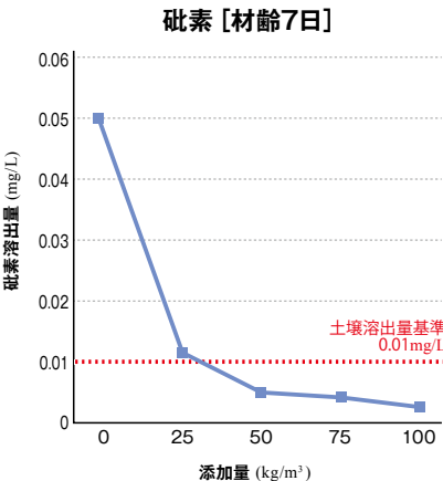
溶出試験
