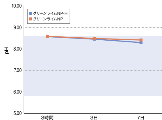
pH 添加量60kg/m³
