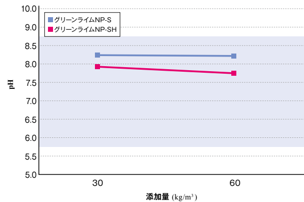
pH 材齢1日
