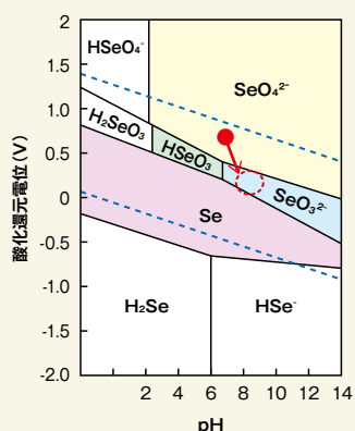
&lt;セレンのpH-酸化還元電位&gt;
