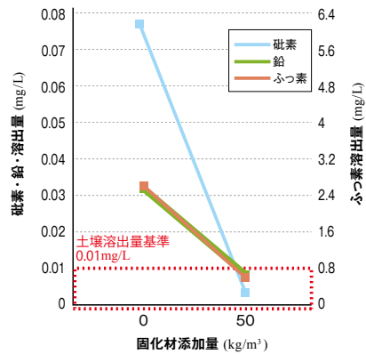
不溶化試験
