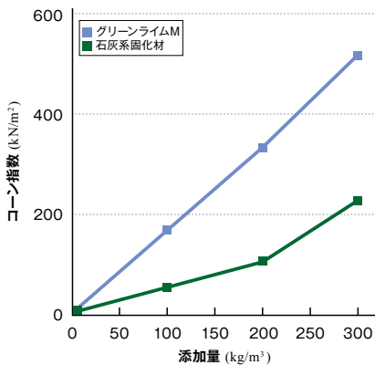
【材齢7日】
