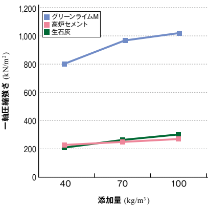
【材齢7日】
