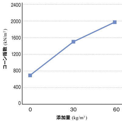
コーン指数試験
