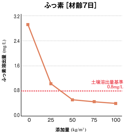
溶出試験
