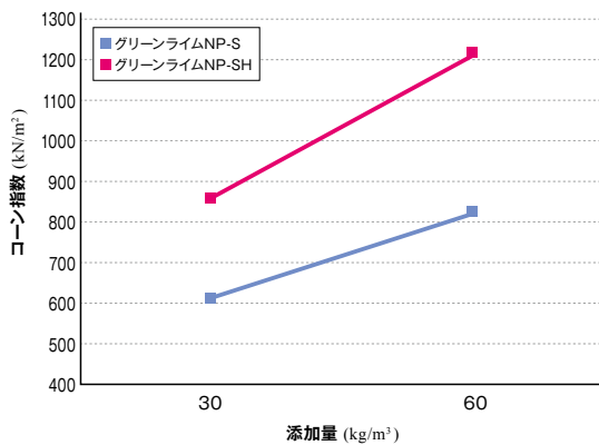
コーン指数 材齢1日
