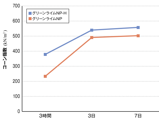
コーン指数 添加量60kg/m³
